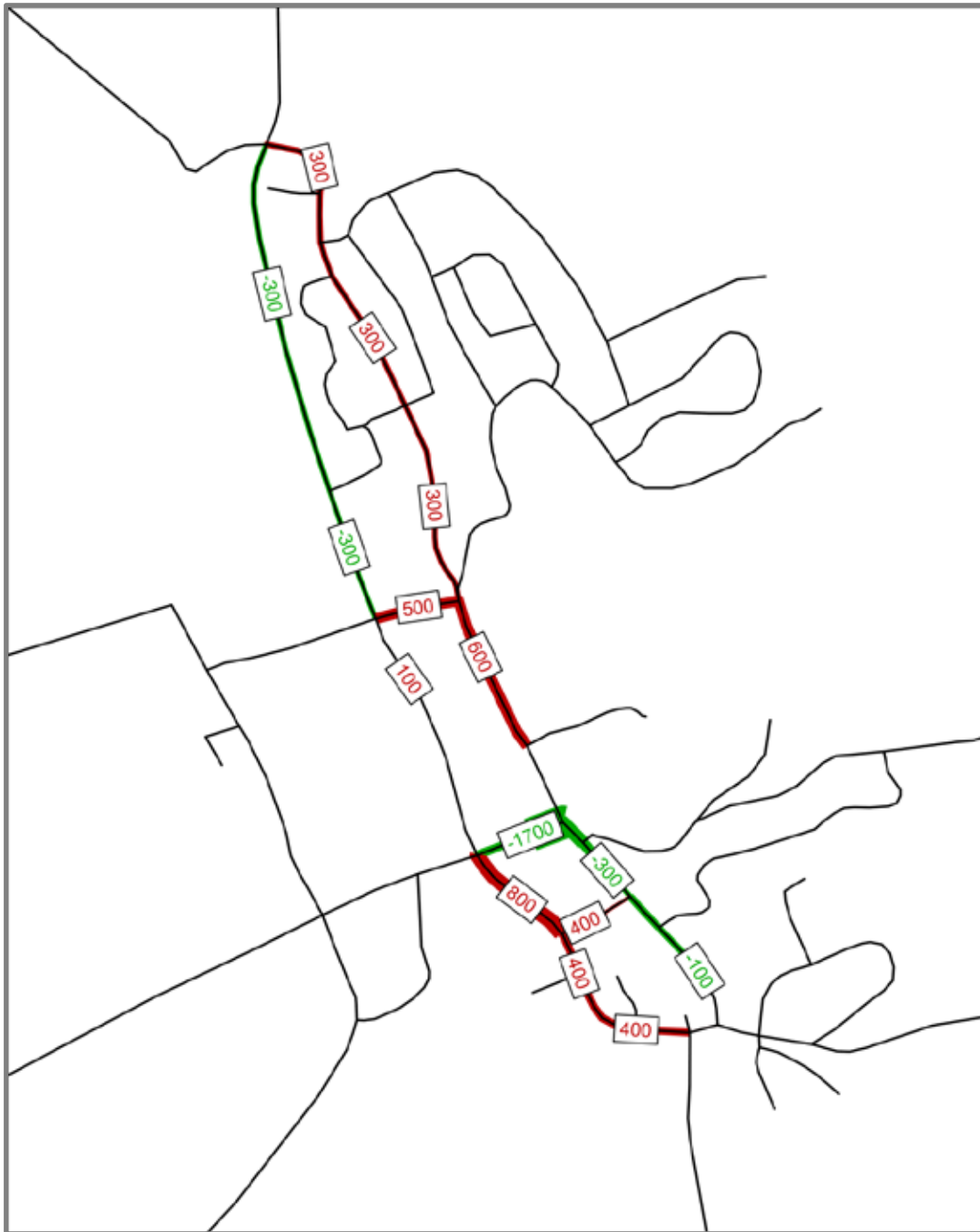
Abbildung 27 Verkehrliche Wirkung einer Sperrung des Marktplatzes im östlichen Bereich für den Kfz-Verkehr [Kfz/ 24h]
