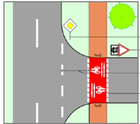
Abbildung 37 Musterlösung für eine hervorgehobene Furt [Ministerium für Verkehr Baden-Württemberg [6]]
