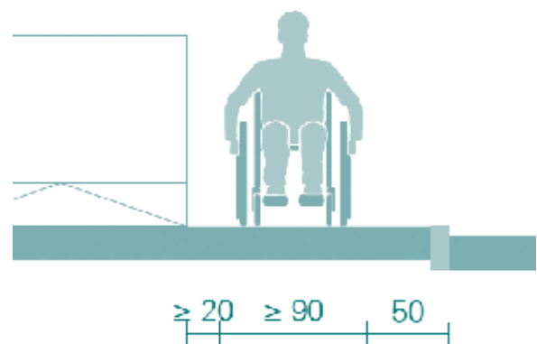
Abmessungen der nutzbaren Gehwegbreite und der Sicherheitsräume bei baulich bedingter Engstelle.
